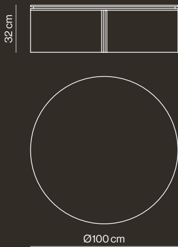
SLOTR-00
