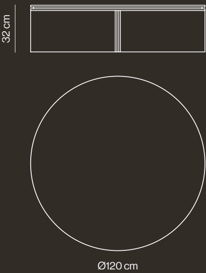
SLOTR-22
